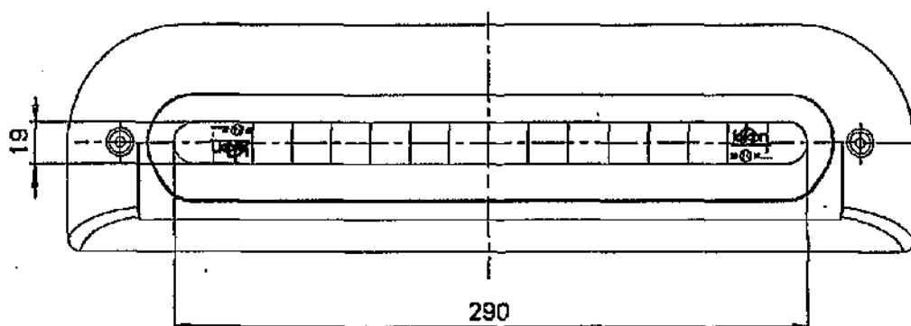
Ansicht von Vorne / front view
